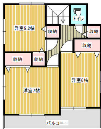
2階平面図
